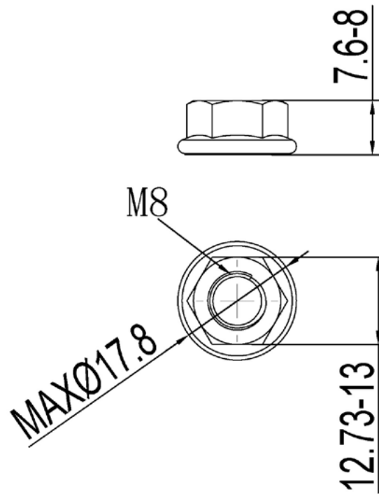
M8 Flange Nut Material: SUS 304
