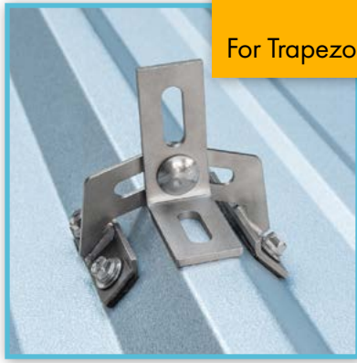
Trapezoidal Rib Metal
